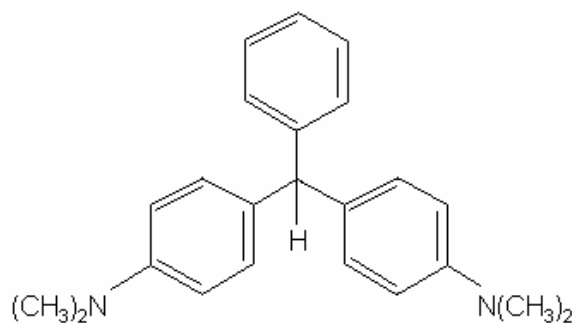
ロイコマラカイトグリーン(Leucomalachite green ; LMG)
