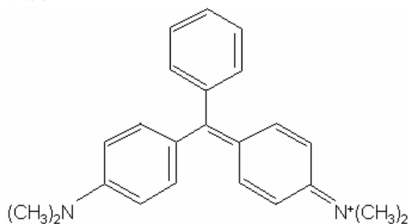
マラカイトグリーン(Malachite green ; MG)
