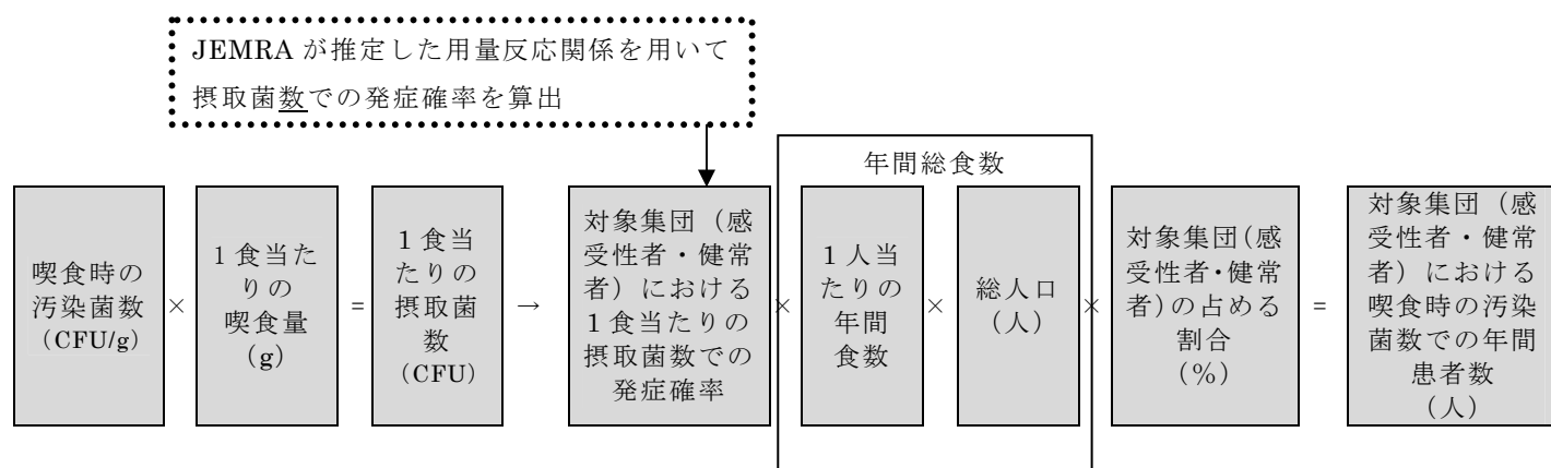
図 11 LM 感染症年間患者数推計手法 概念図
