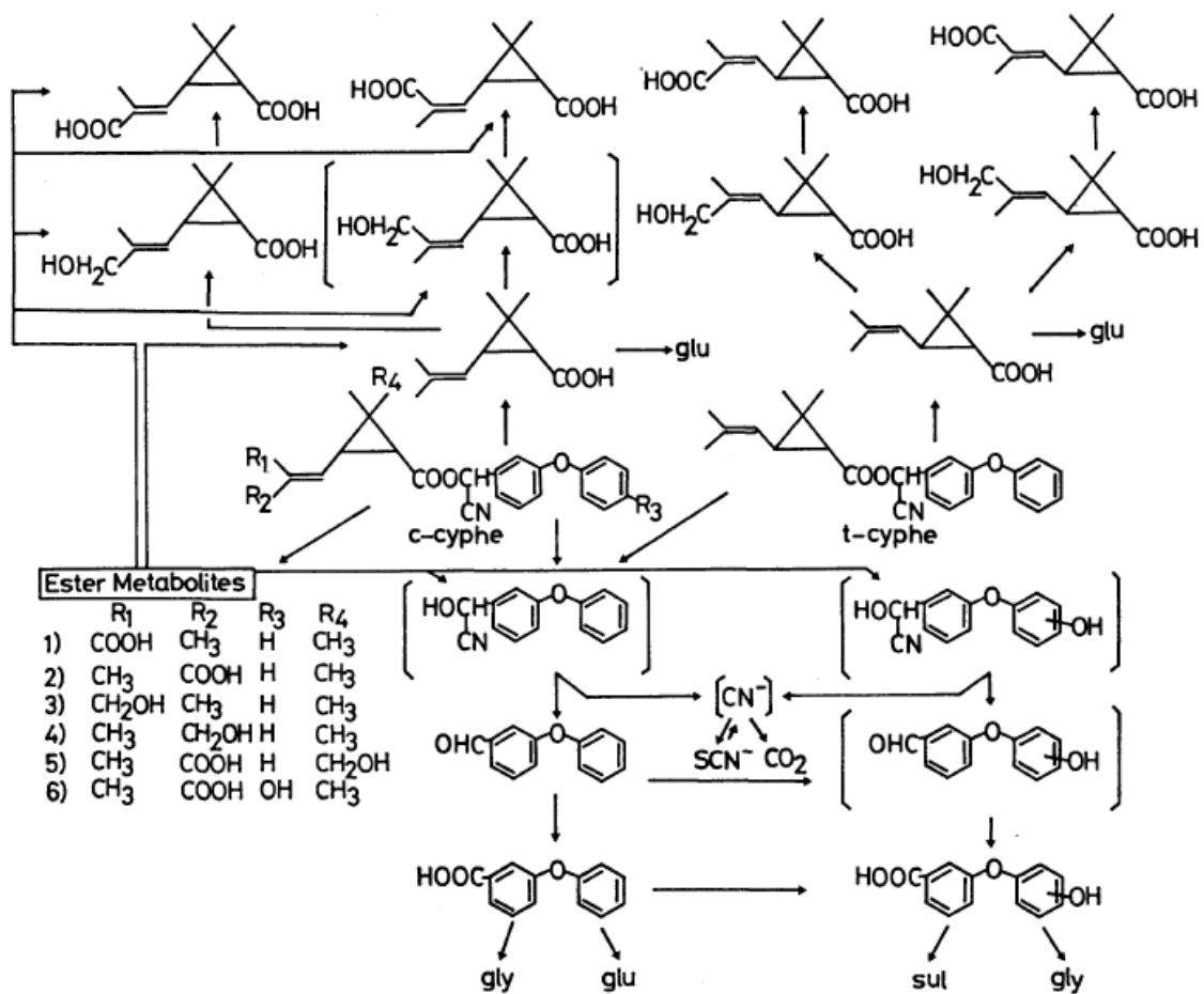
図2 \alpha T80-シフェノトリン ([1R]シス体又は[1R]トランス体) のラットにおける推定代謝経路 (参照8)
