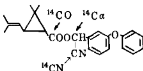
図 1 ^{14}\text{C} 標識体の標識位置
