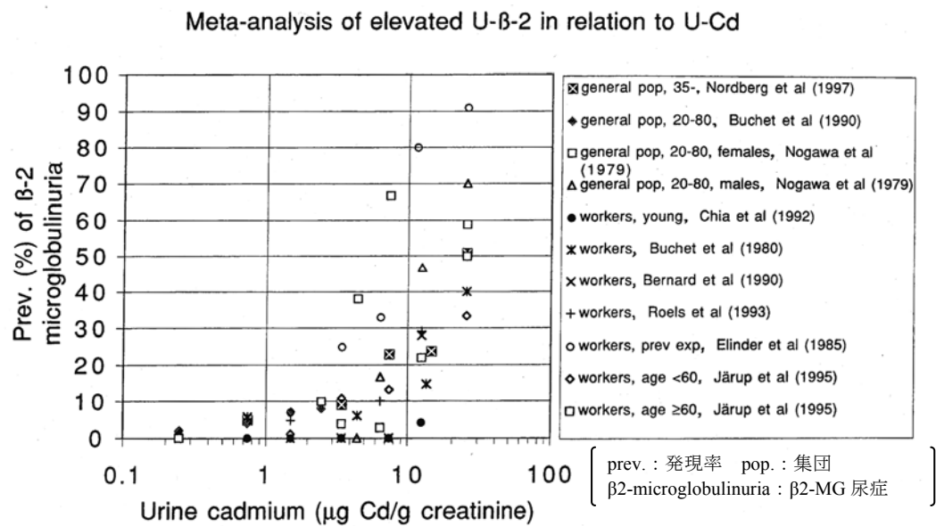
図1 尿中カドミウム排泄量と尿中 \beta 2-MG 排泄量の上昇に関するメタアナリシス
