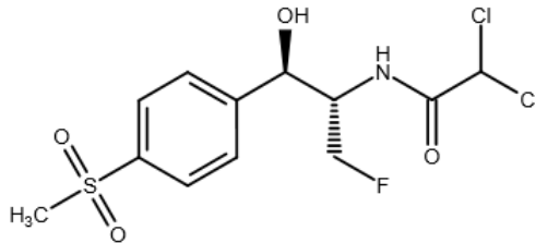
フロルフェニコールの構造式
