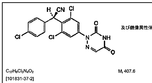
ジクラズリルの構造式
