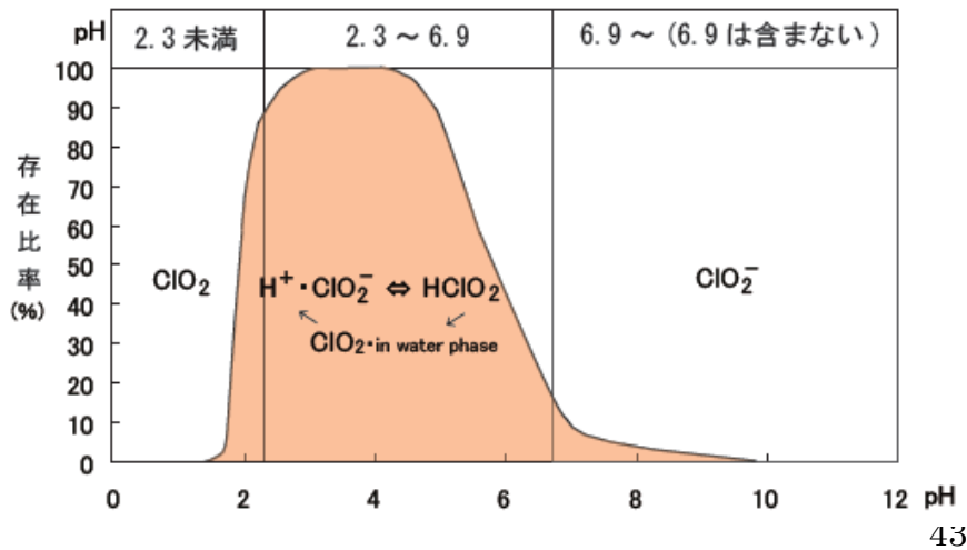
図-1 亜塩素酸水に含有する塩素酸化物のpHによる存在比の変化(事業者提供資料より)
