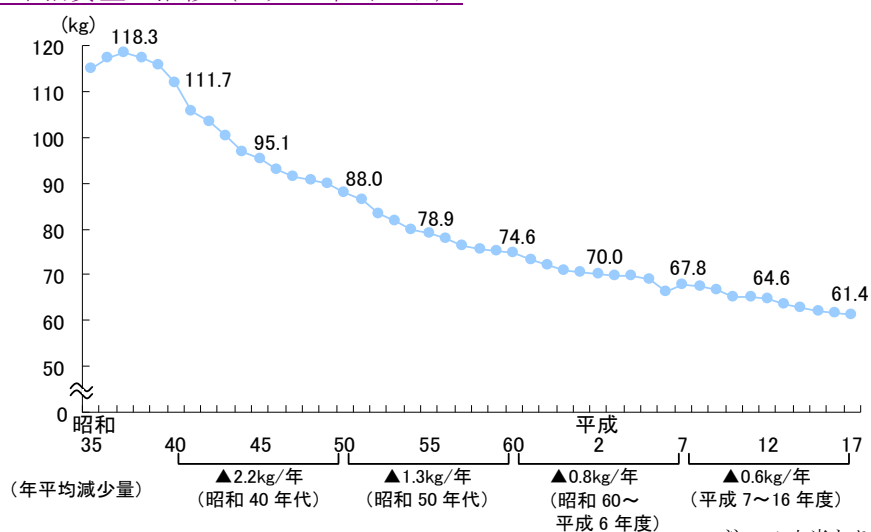
32 図 14 米消費量の推移(1人1年当たり)
