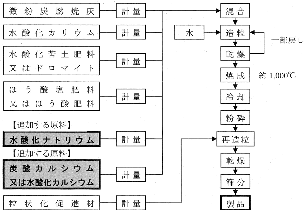
図 1 製造工程の概要
