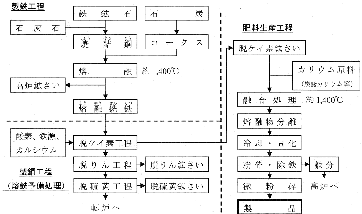
図 2 製造工程の概要
