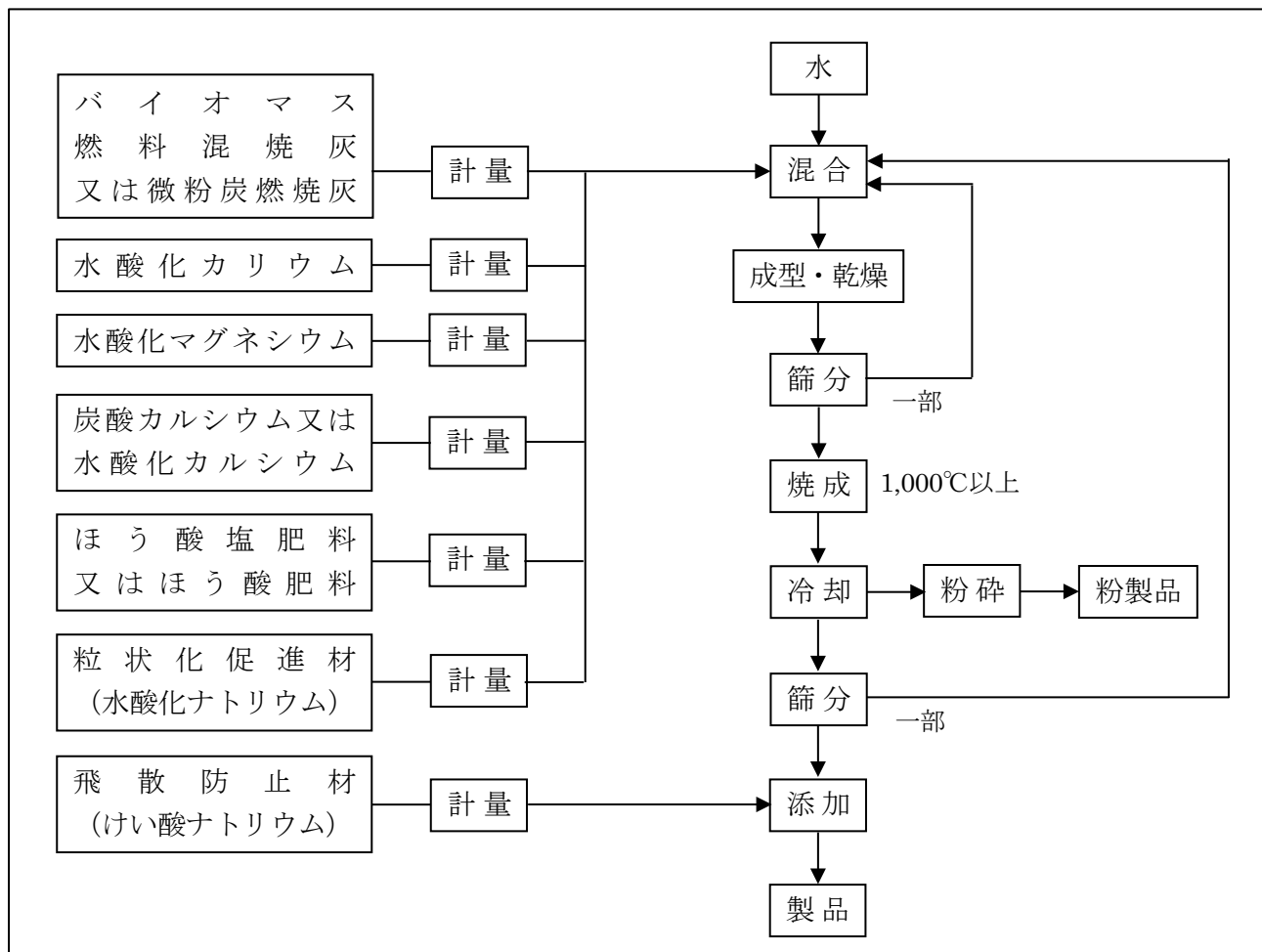
図 1 生産工程の概要
