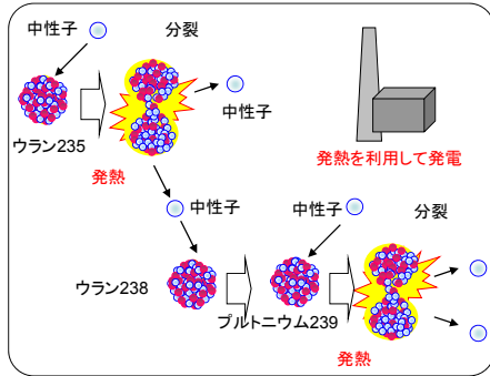
原子炉内部での反応
