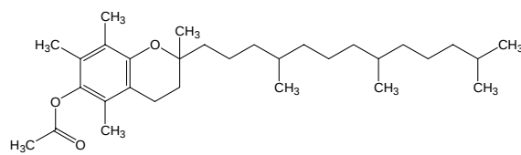
酢酸 dl - \alpha -トコフェロール
