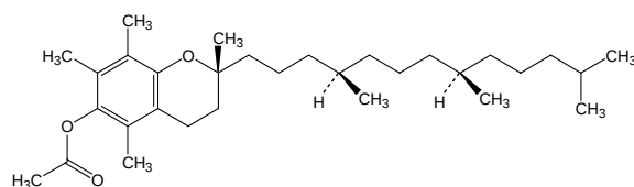
酢酸 d - \alpha -トコフェロール
