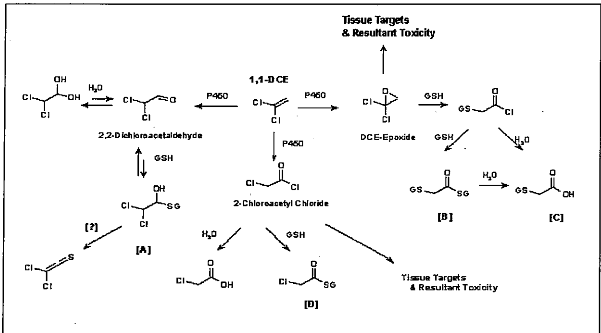
図 1. 1,1-DCE の代謝経路 (Forkert 1999a 8 , CICAD 2003 2 )
