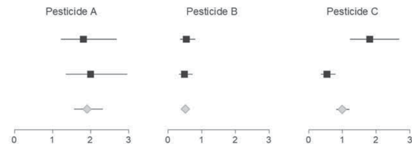
図 1.3 3 つの農薬 (A、B、C) のそれぞれが 2 つの研究のメタアナリシスで評価されている仮想例のフォレストプロット。各プロットの x 軸は、ばく露した個体とばく露していない個体を比較した、対象疾患の推定リスク比を表している。四角は各研究における推定リスク比を示し、灰色のダイヤモンドは要約されたリスク比を示している。横線は 95% 信頼区間を示す。
