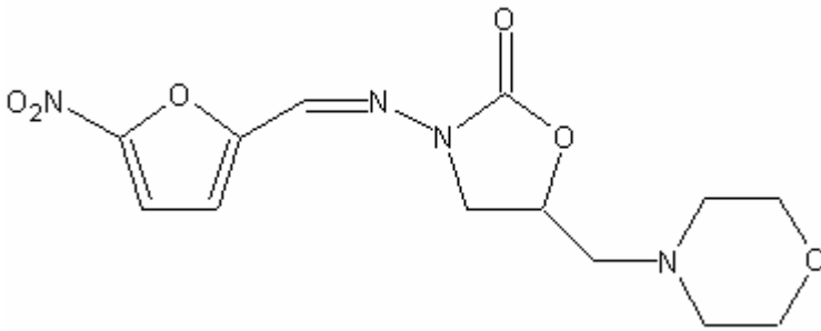
16 フラルタドン
