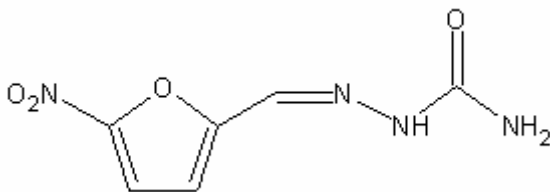
36 ニトロフラゾン
