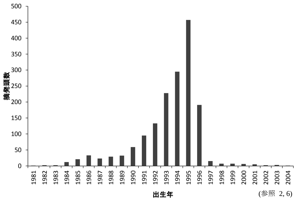
図3 アイルランドの出生年別のBSE検査陽性牛頭数
