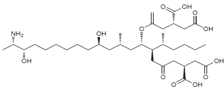
Fumonisin B 3
