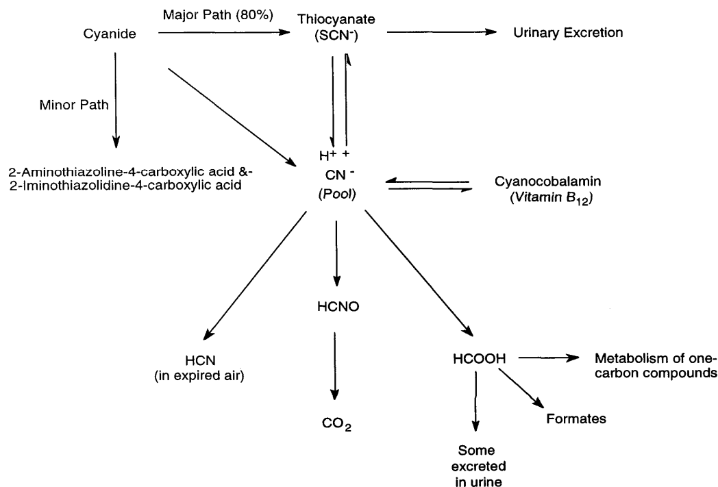
図 シアン化物の基本的代謝経路 (参照 3, 3a)
